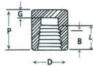
Cap
