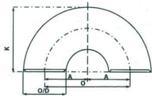
180 Deg. LR RETURN BEND
